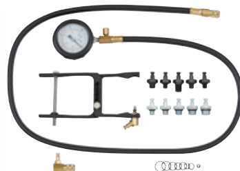
#818011 Oliedruk-testset, 14-dlg.
